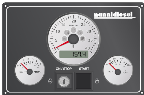
Nanni C4 paneel
